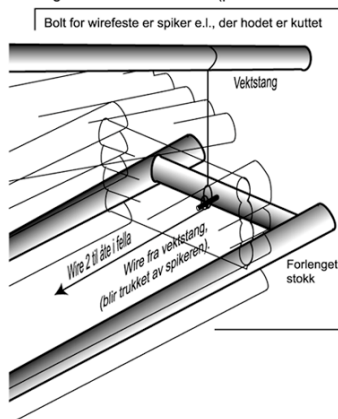
Fig 4. Utløsermekanisme (på fellas bakkant)
