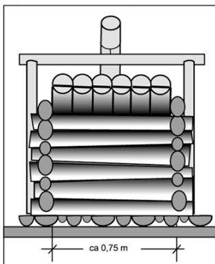
Fig 3. Fellefront m/lokket åpent
